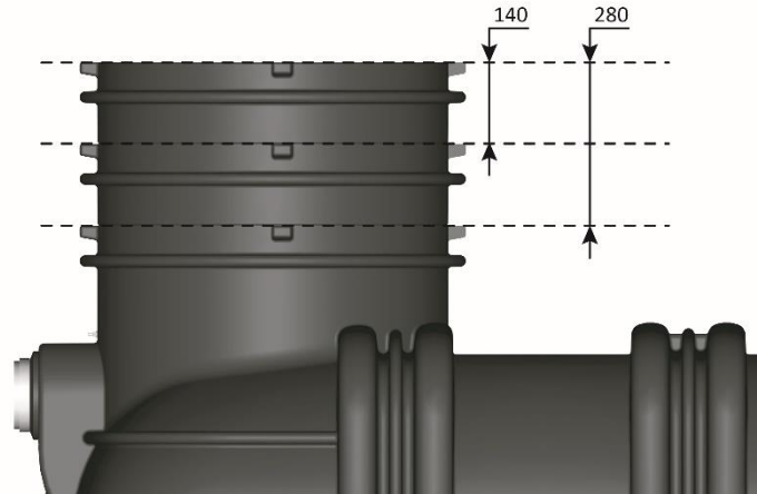
Niveau de découpe possibles des réhausses intégrées (exemple de la réhausse intégrée sur l'accès en DN 600 de l'unité de traitement primaire)
