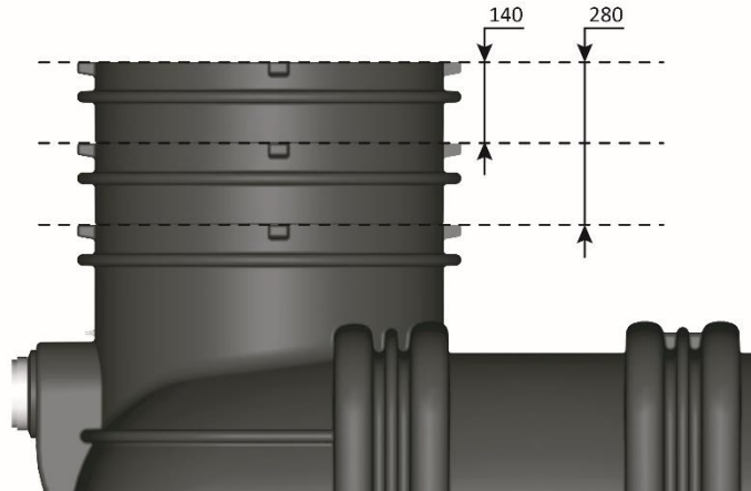
Niveau de découpe possibles des rehausses intégrées (exemple de la rehausse intégrée sur l'accès en DN 600 de l'unité de traitement primaire)
